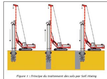
Figure 1 : Principe du traitement des sols par Soil Mixing
